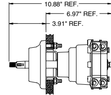
90DEG. BEZEL MOUNTING ( SB 27150 )
