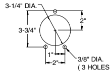
90DEG. BEZEL
